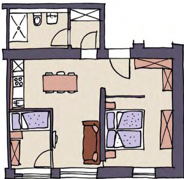
Beispielgrundriss 2 Zimmer
